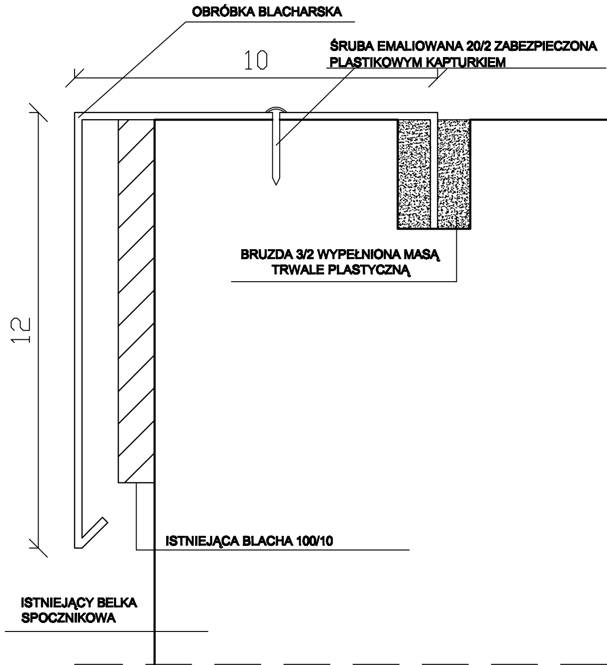
PRZEKRÓJ 1:1
